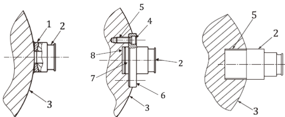
a) 焊接耳轴
